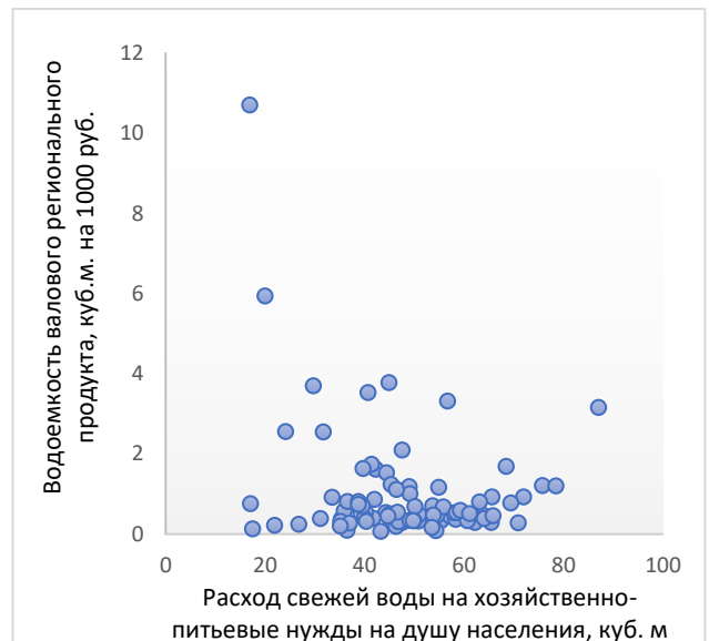
Рисунок 20. Водоемкость ВРП и удельное бытовое водопотребление
